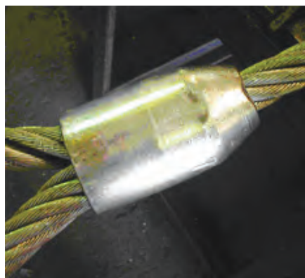
Втулка, опрессованная в наружной полости матрицы
