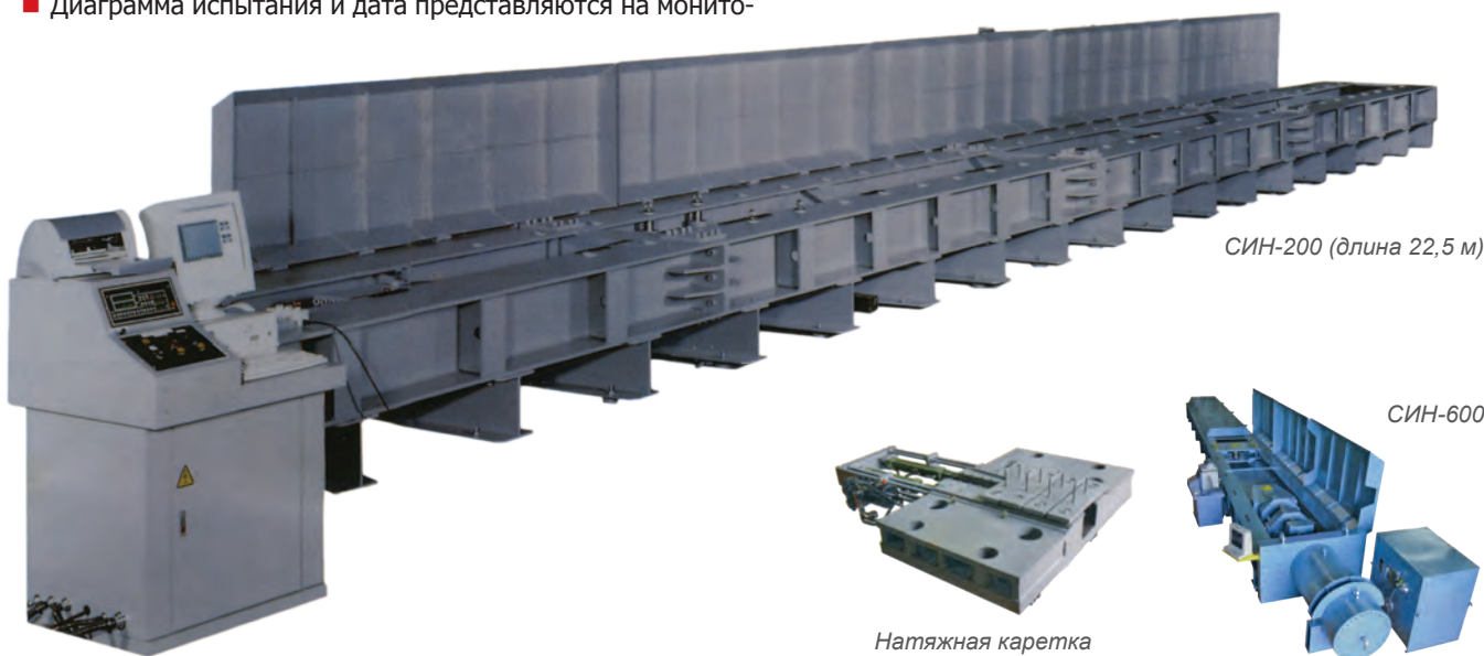
Технические характеристики стендов гидравлических, серии «ADVANCED»
